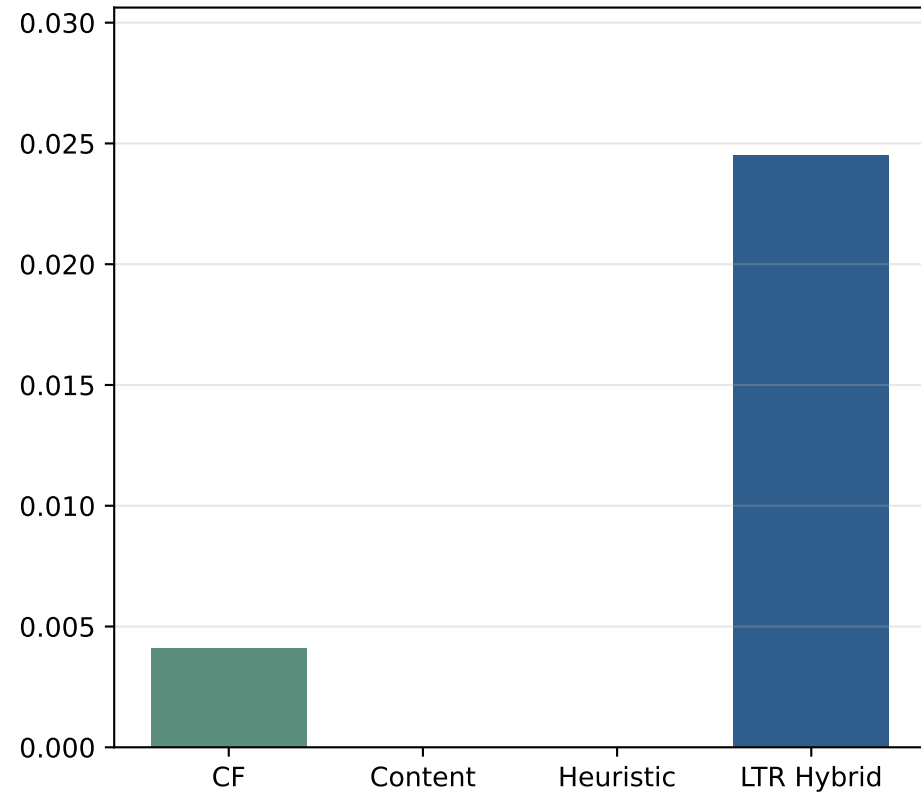
Precision@5
